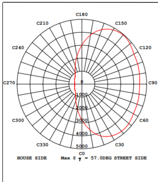
DIAGRAMA DE DISTRIBUCIÓN DEL ESPACIO CÓNICO DE INTENSIDAD MÁXIMA
