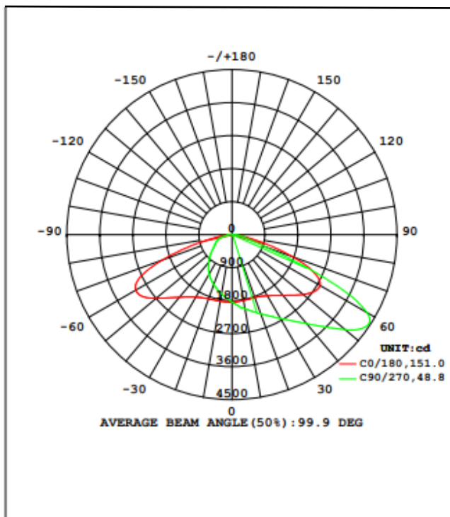
DIAGRAMA DE DISTRIBUCIÓN DE LA INTENSIDAD EN PLANOS C
